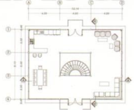
نقشه مبلمان طبقه همکف Furniture plan, ground floor
