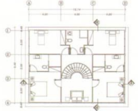
نقشه مبلمان طبقه زیرزمین ۱- Furniture plan, -1 basement floor
